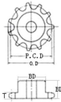
东正双节距链轮参数
